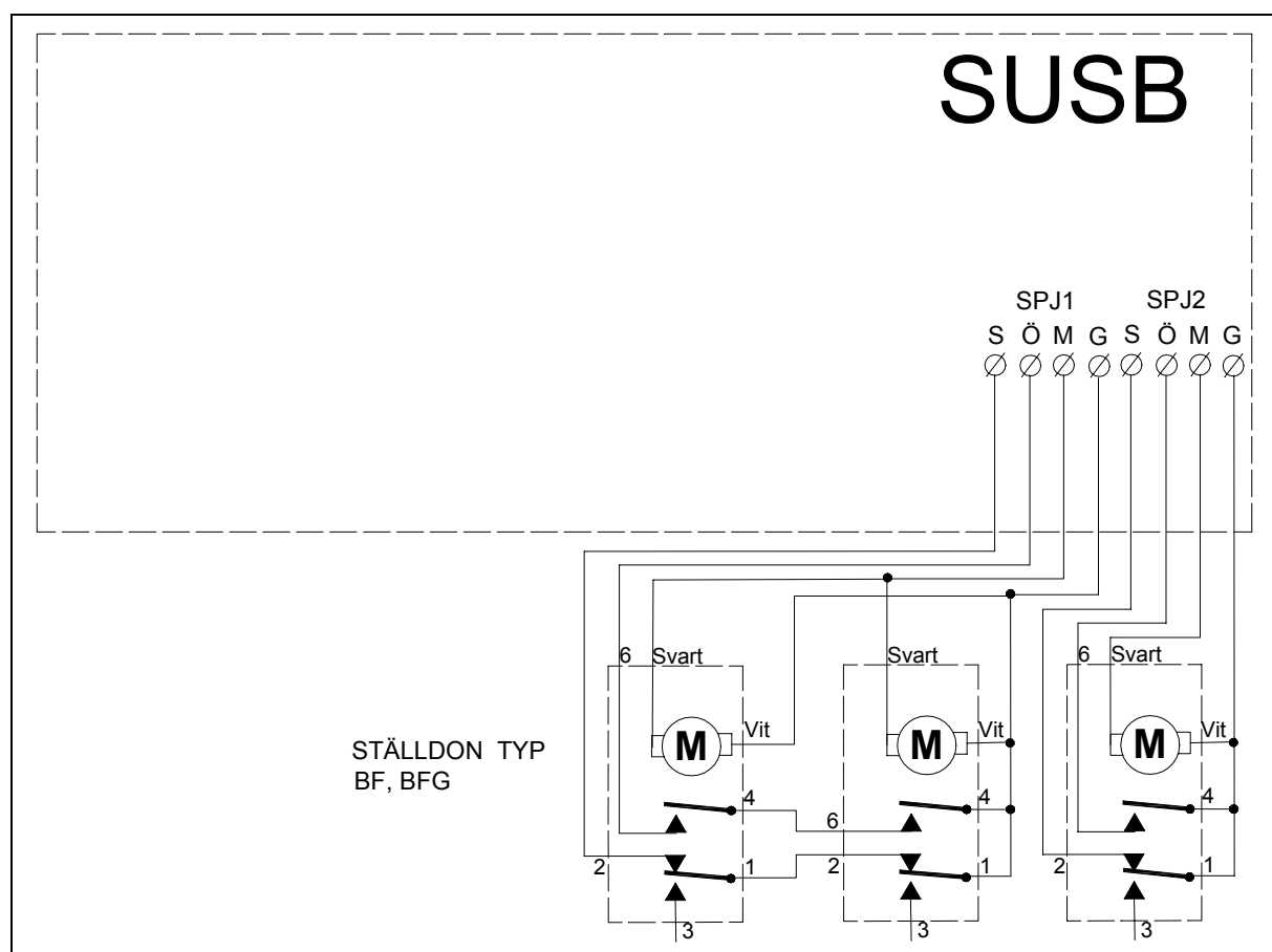
Bild utvisande parallellkoppling på spjällgrupp 1 och enkelt spjäll på spjällgrupp 2
